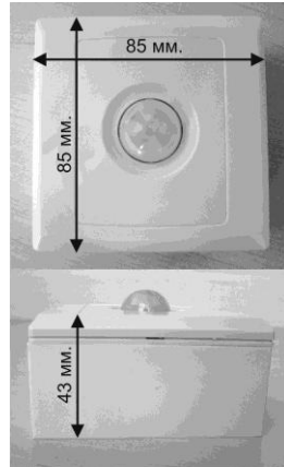
Габариты
