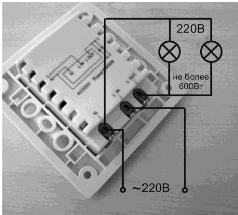
Схема подключения
